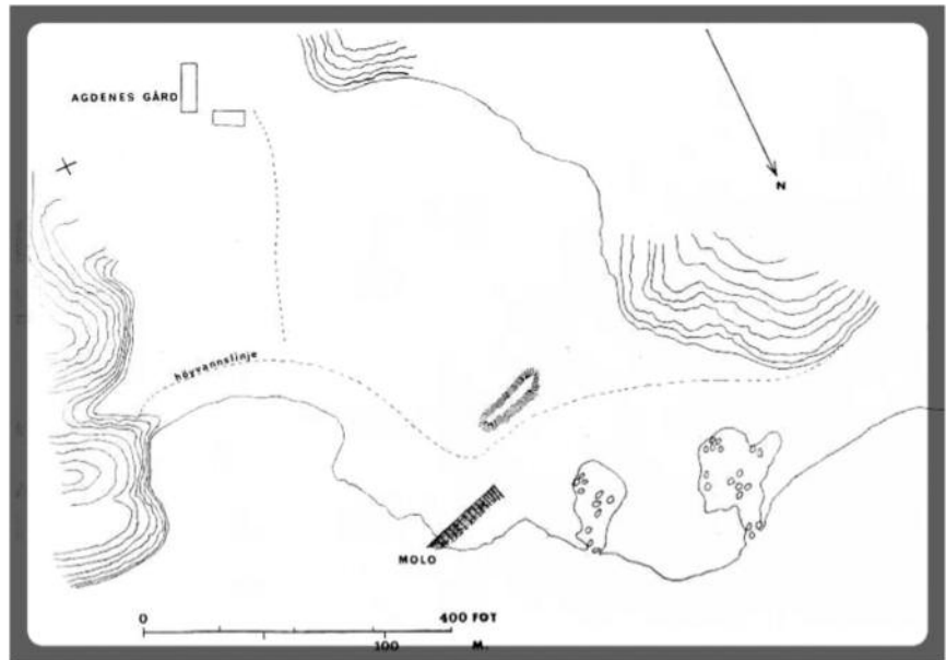
Ingeniør J Meyers kart over restene av havneanlegget på Agdenes gård etter befaringen i 1869.
